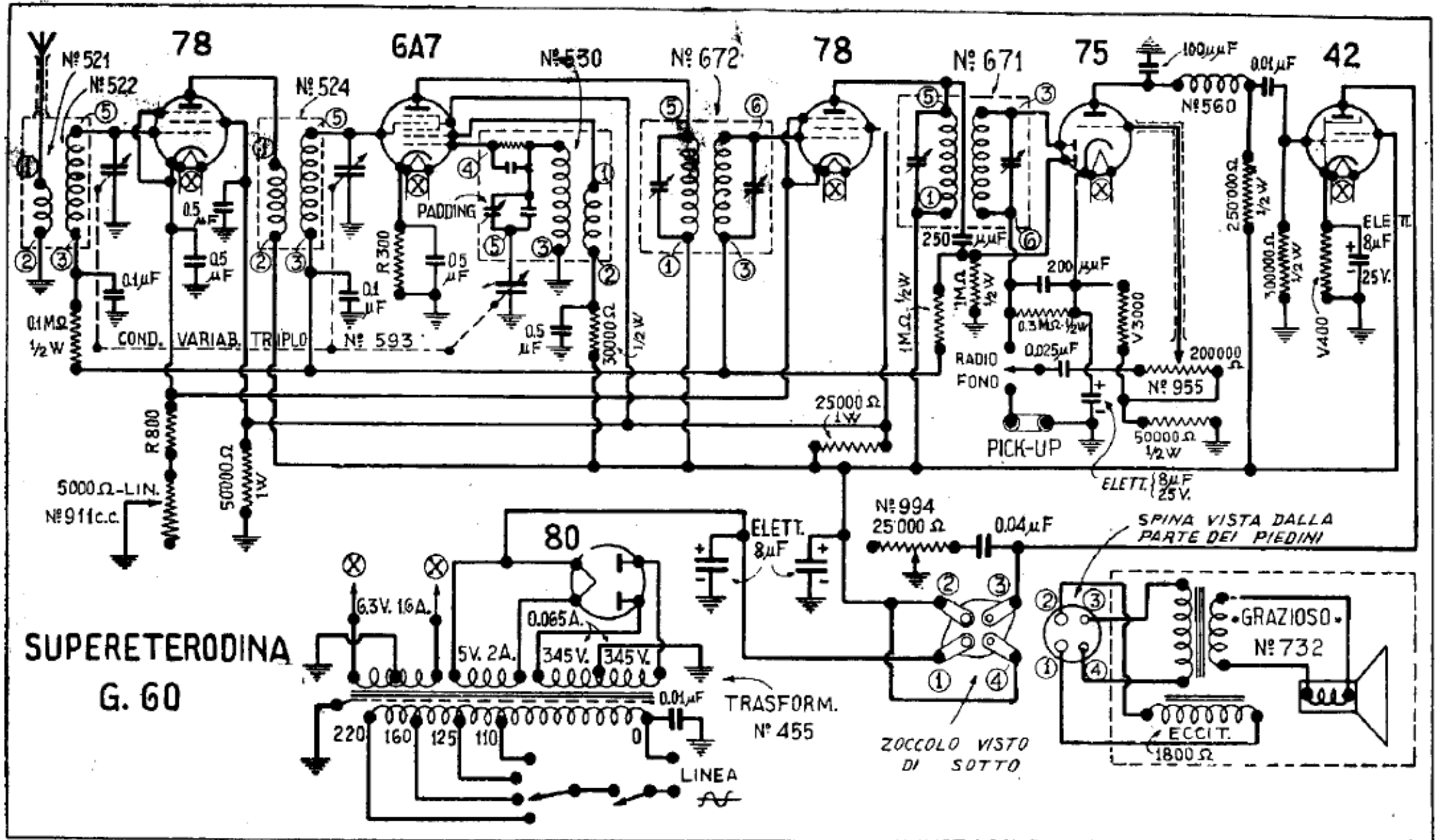
• Lo schema elettrico della Super G-60.
